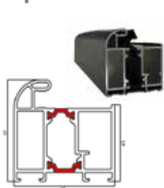
Ościeżnica TERMO
