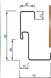
Ościeżnica „9”
