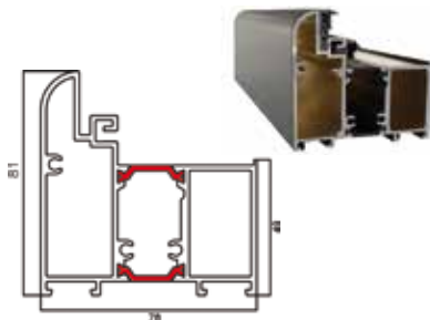
Ościeżnica TERMO PRESTIGE
